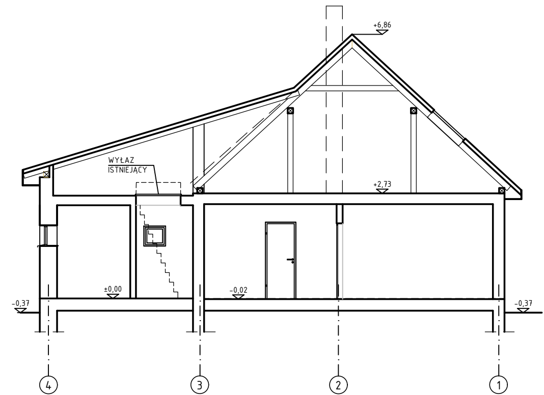
PRZEKRÓJ A-A, 1:100
