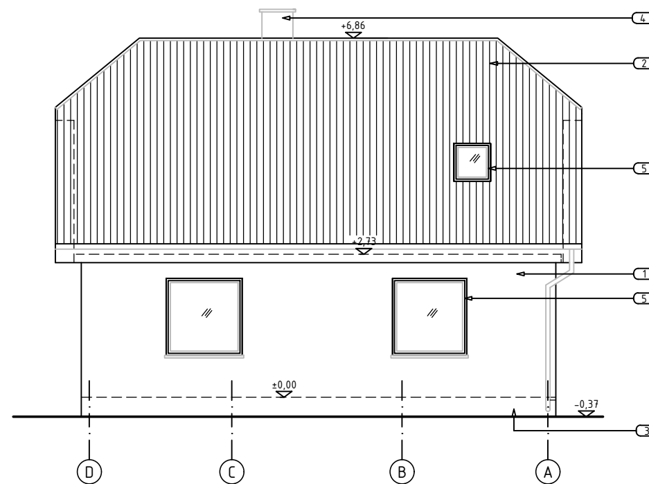
ELEWACJA PÓŁNOCNA, 1:100
