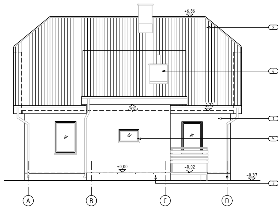
ELEWACJA POŁUDNIOWA, 1:100
