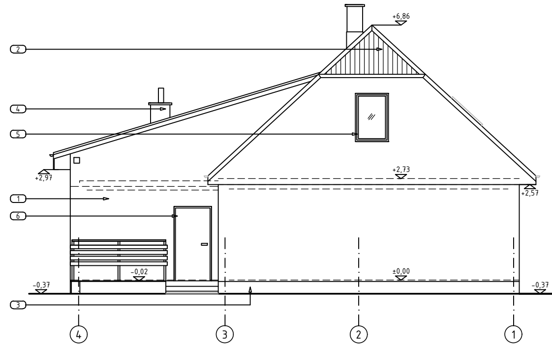
ELEWACJA POŁUDNIOWA, 1:100
