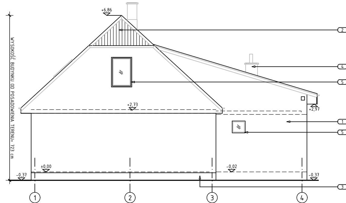
ELEWACJA PÓŁNOCNA, 1:100
